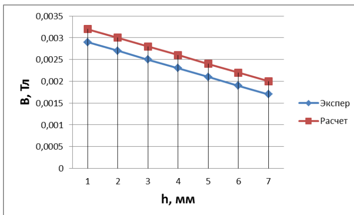
Рис. 2. Изменение величины магнитной индукции над головкой рельса
